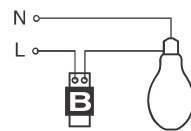
วงจรการต่อใช้งาน สำหรับหลอดไอปรอทความดันสูง
